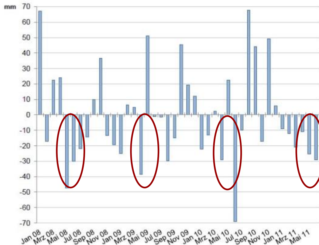
Abb. 13: Abweichung des Monatsniederschlags zum langjährigen Mittel im Zeitraum von Januar 2008 bis Juni 2011 (aus METEOROLOGISCHES INSTITUT 2011, verändert)
