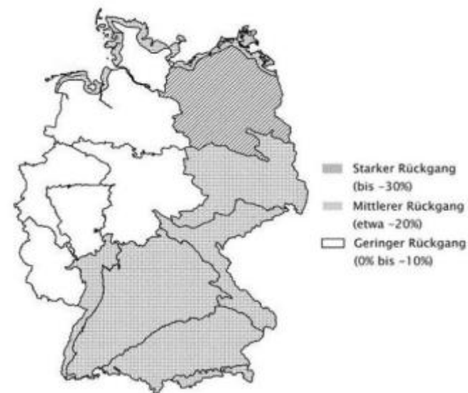
Abb. 10: Prognosen für die Niederschlagsänderung im Sommer (2071 - 2100 minus 1961 - 1990) (aus SPEKAT 2007, Anhang H)
